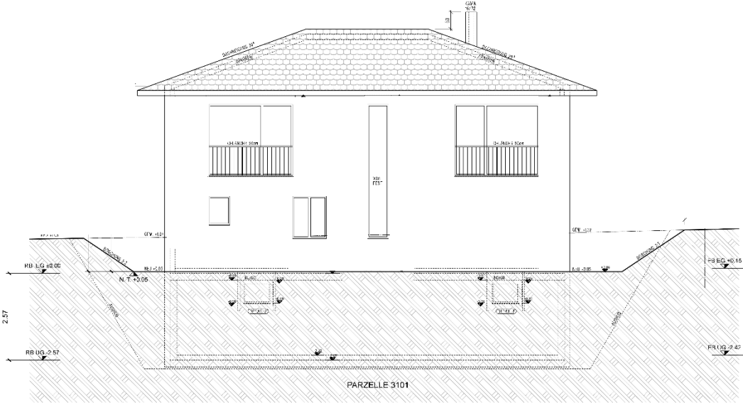
Nordfassade
