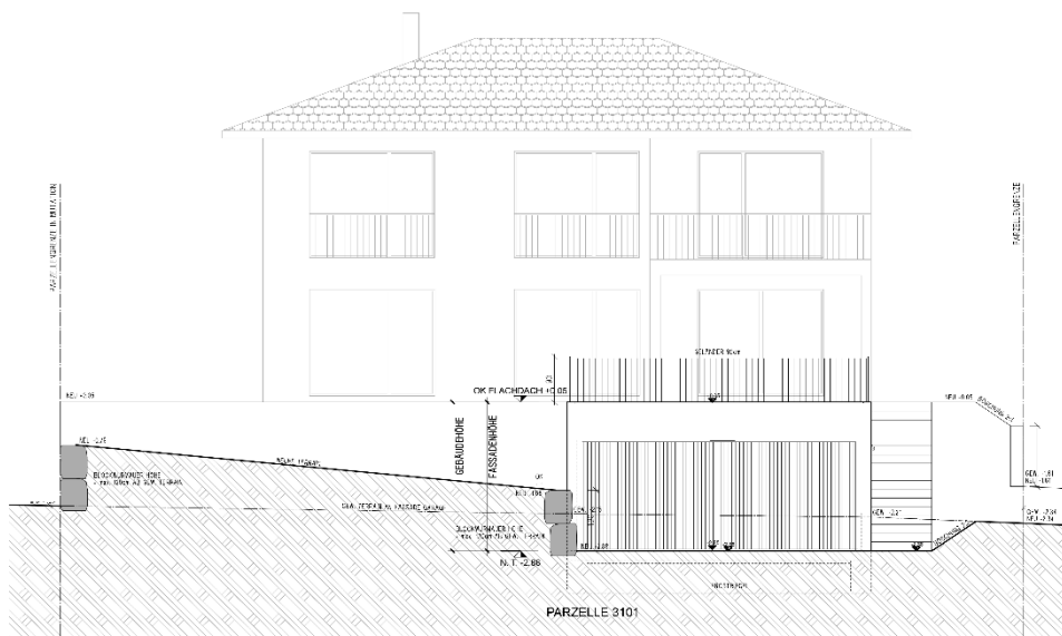
Südfassade
