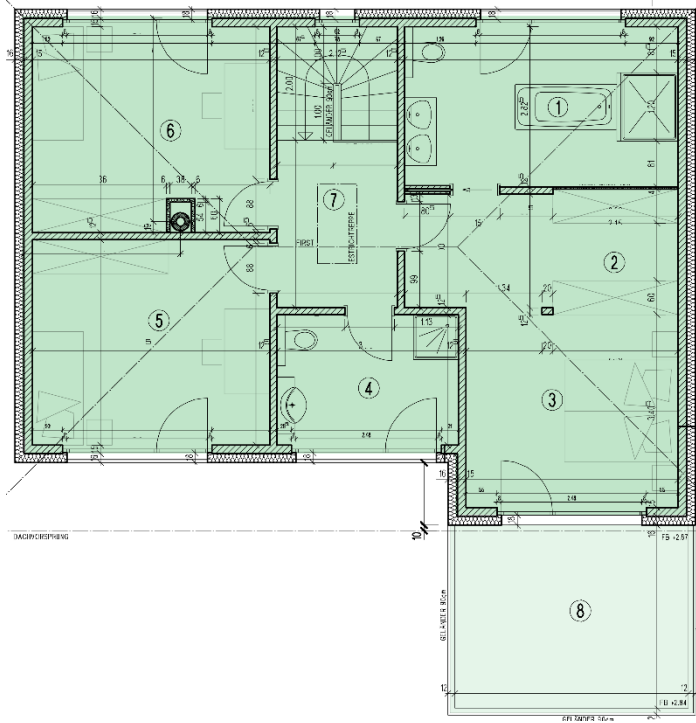
Dachgeschoss
