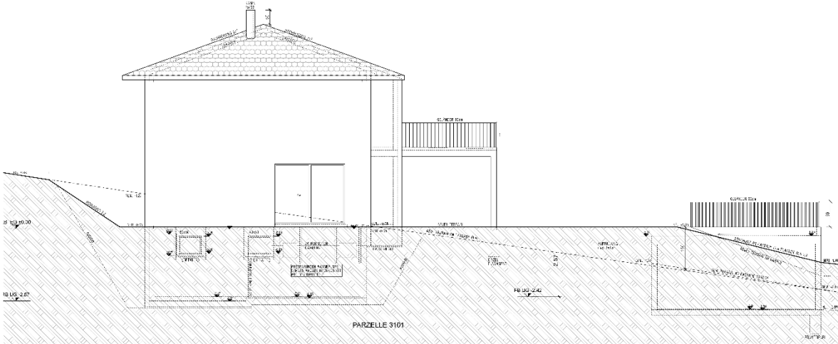
Westfassade
