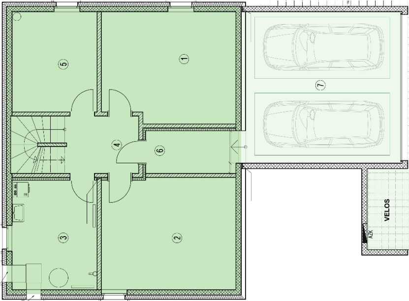
Untergeschoss
