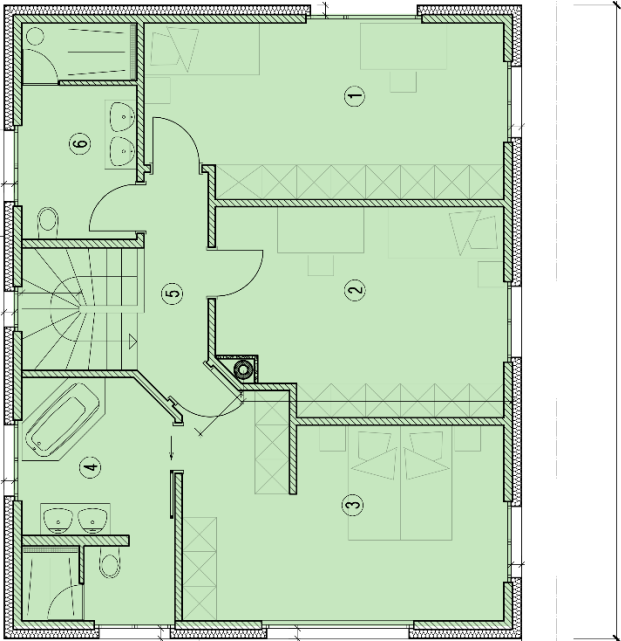
Dachgeschoss
